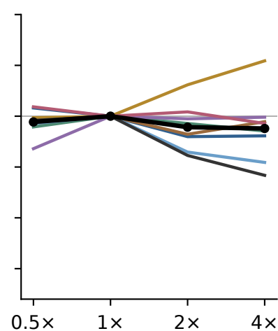
\lambda_{\text{mod}}
