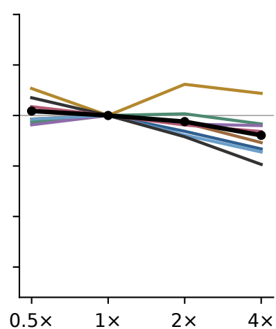
\lambda_{\text{nbr}}
