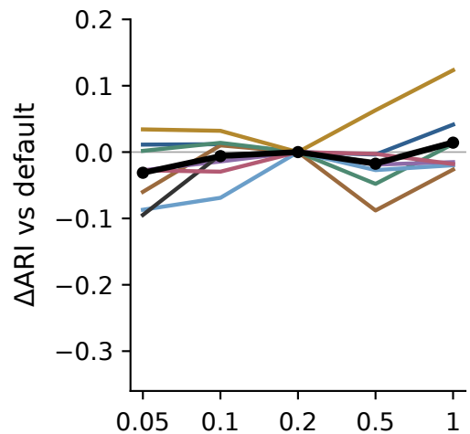
\tau_e
