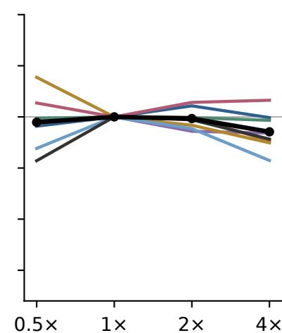
\lambda_{\text{sm}}
